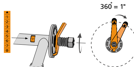
2. Otočte klikou o jednu otáčku a nastavte pilový řez na prkno o tloušťce 1 palce.
