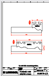
Exempel på ritning av specialprofilstål.
