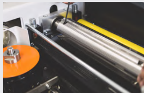
Stora tandade matarvalsar och gummerad utmatningsvals för att skydda den fint hyvlade ytan.
