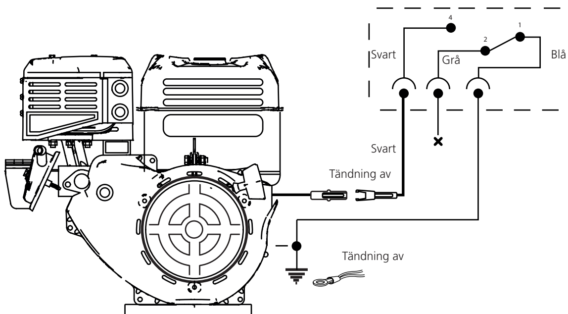
Säkerhetsbrytare
